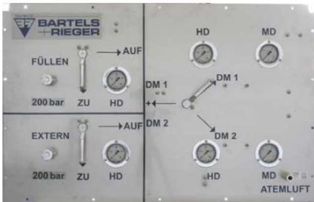
Bedienpult des Atemschatz Containers
